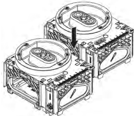
Kopplingsschema
