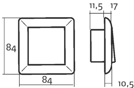
Måttritning
