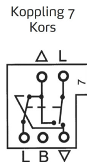
Kopplingsschema
