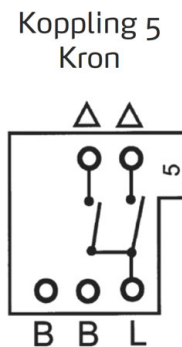
Kopplingsschema
