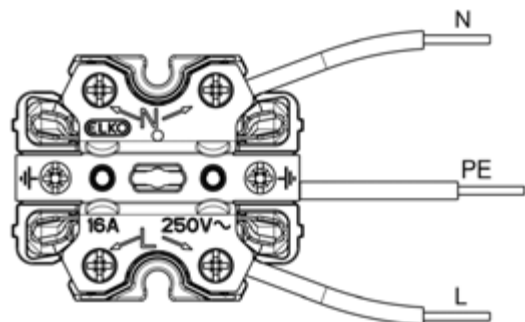
Kopplingsschema
