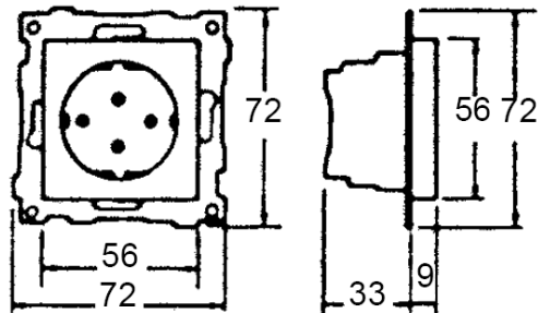
Måttitning
