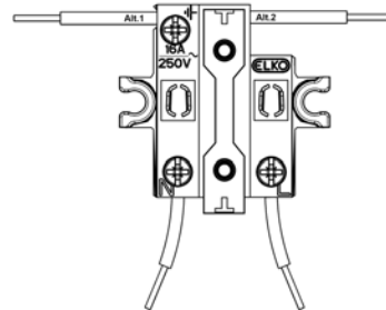
Kopplingsschema
