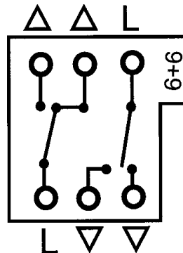
Kopplingsschema
