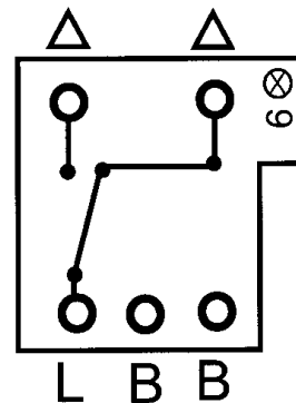
Kopplingsschema
