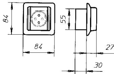
Måttritning
