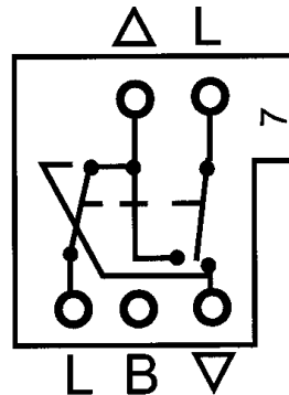
Kopplingsschema
