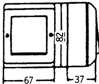
Måttritning
