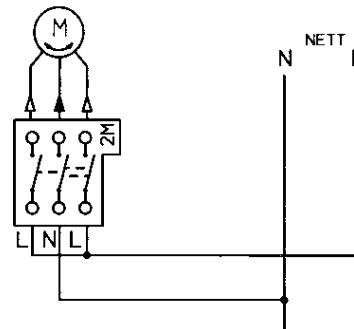
Kopplingsschema
