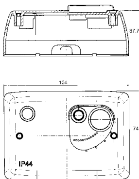
Måttritning
