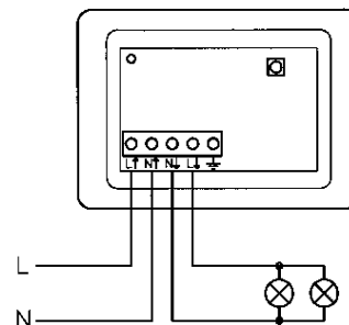
Kopplingsschema
