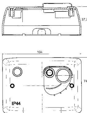
Måttritning
