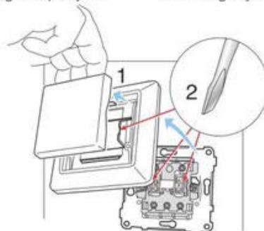
Montering av impulsfjäder.
